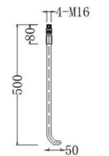
Perno de Anclaje
